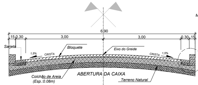
SEÇÃO TRANSVERSAL
