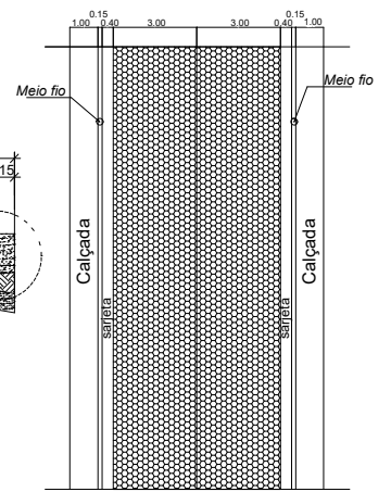
DETALHE DO PAVIMENTO EM BLOQUETE
